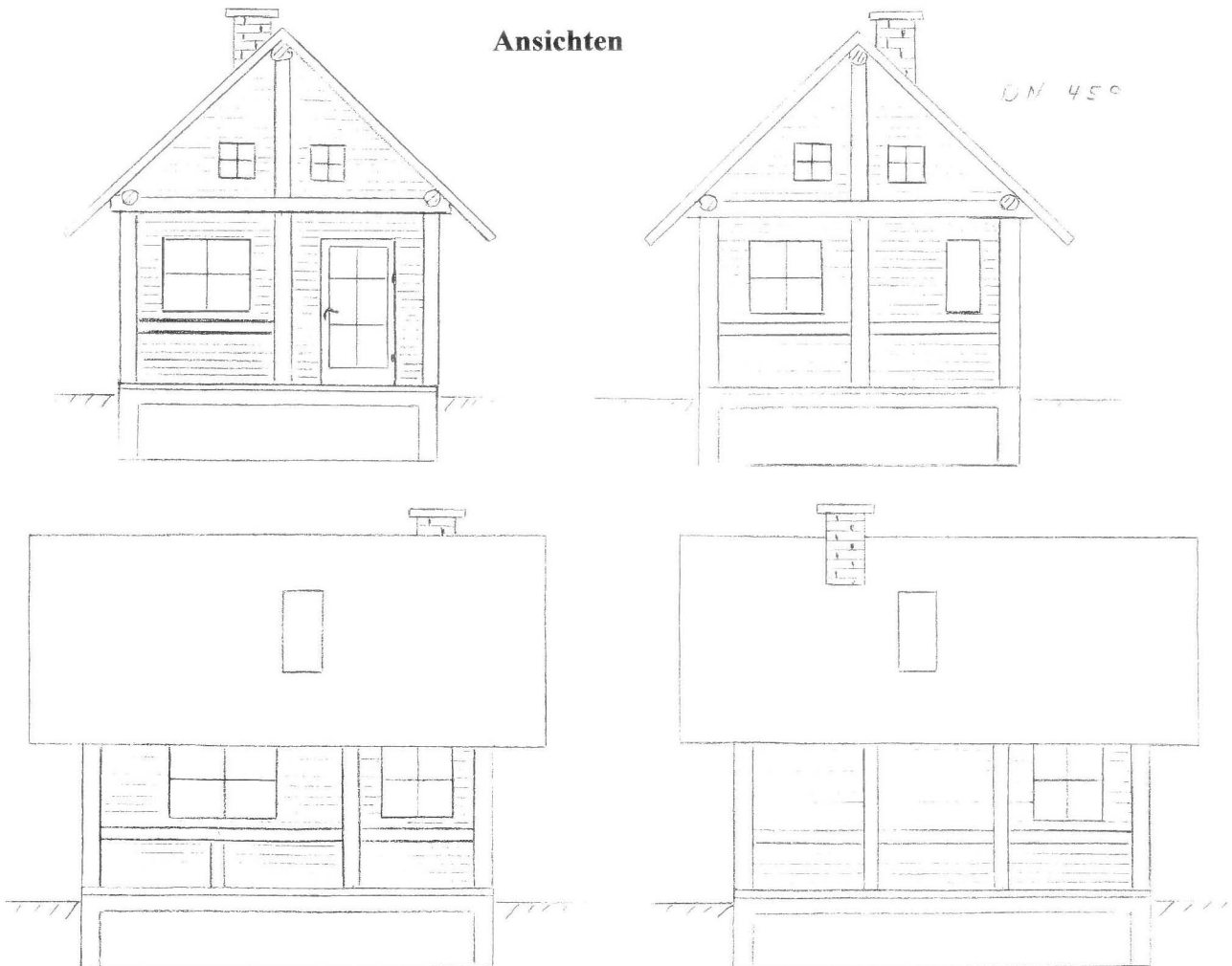
Maßstab 1:100
